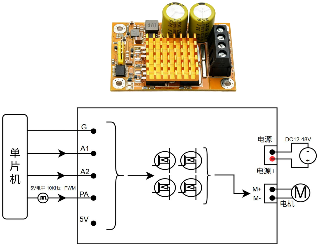
BRT-HDC-30A款驱动器电气连接图
